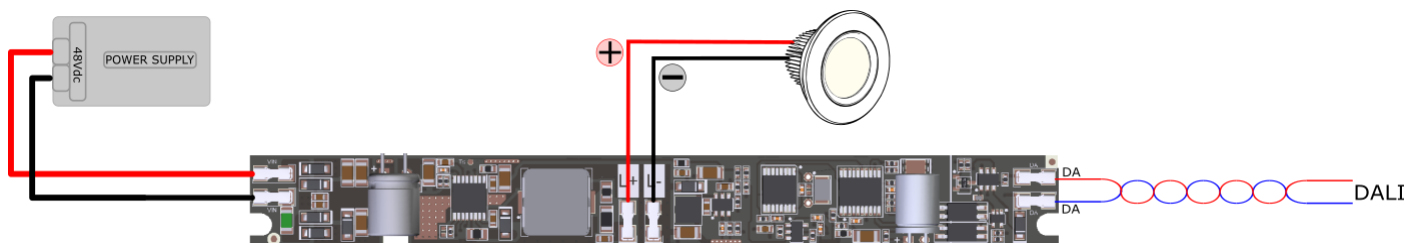
Figura 2: Schema di cablaggio per carichi LED bianchi o monocolori
