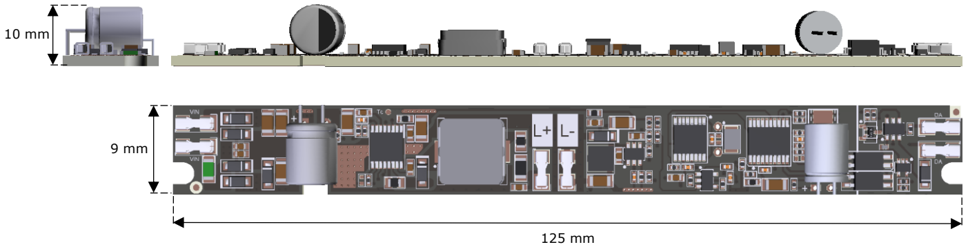
Figura 9: Dimensioni meccaniche
