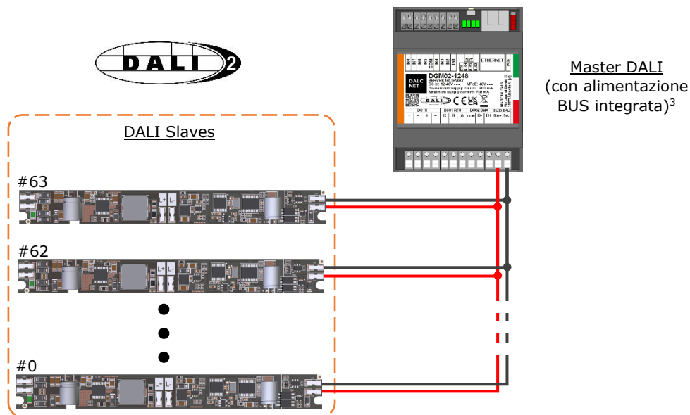
Figura 3: Topologia di connessione del controllo remoto, cablaggio bus
