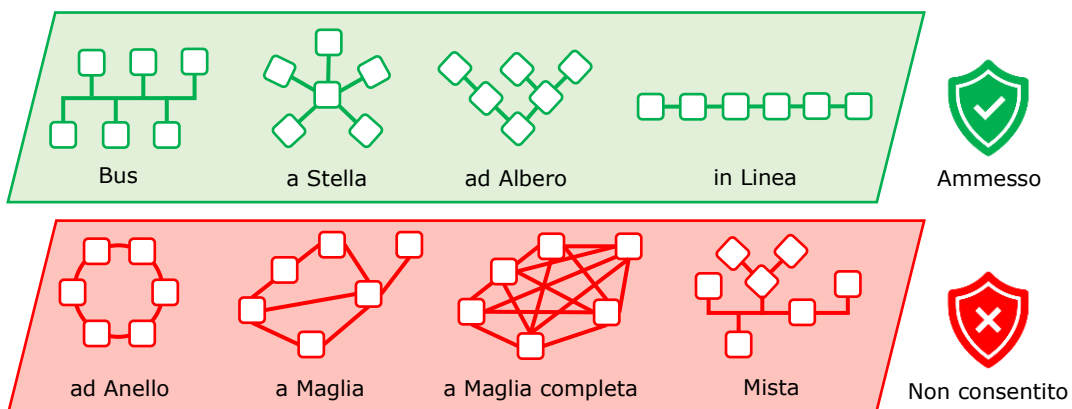
Figura 4: Topologie di cablaggio DALI
