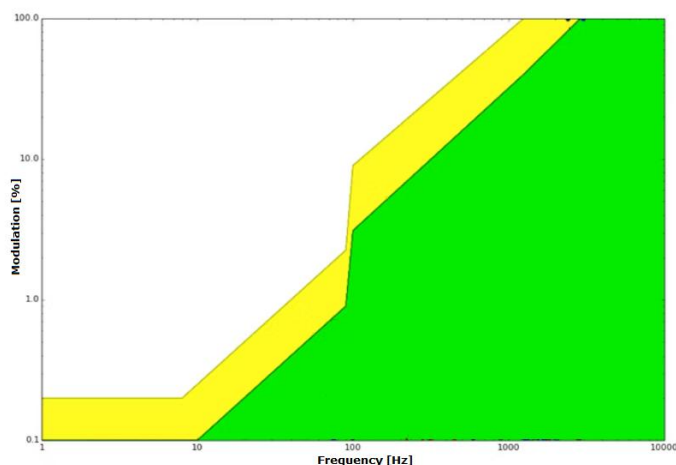
Figura 6: Soglia di percezione dello sfarfallio
